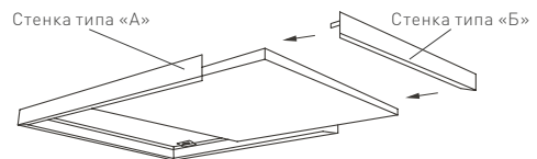
Рис. 4. Установка светильника в рамку.
